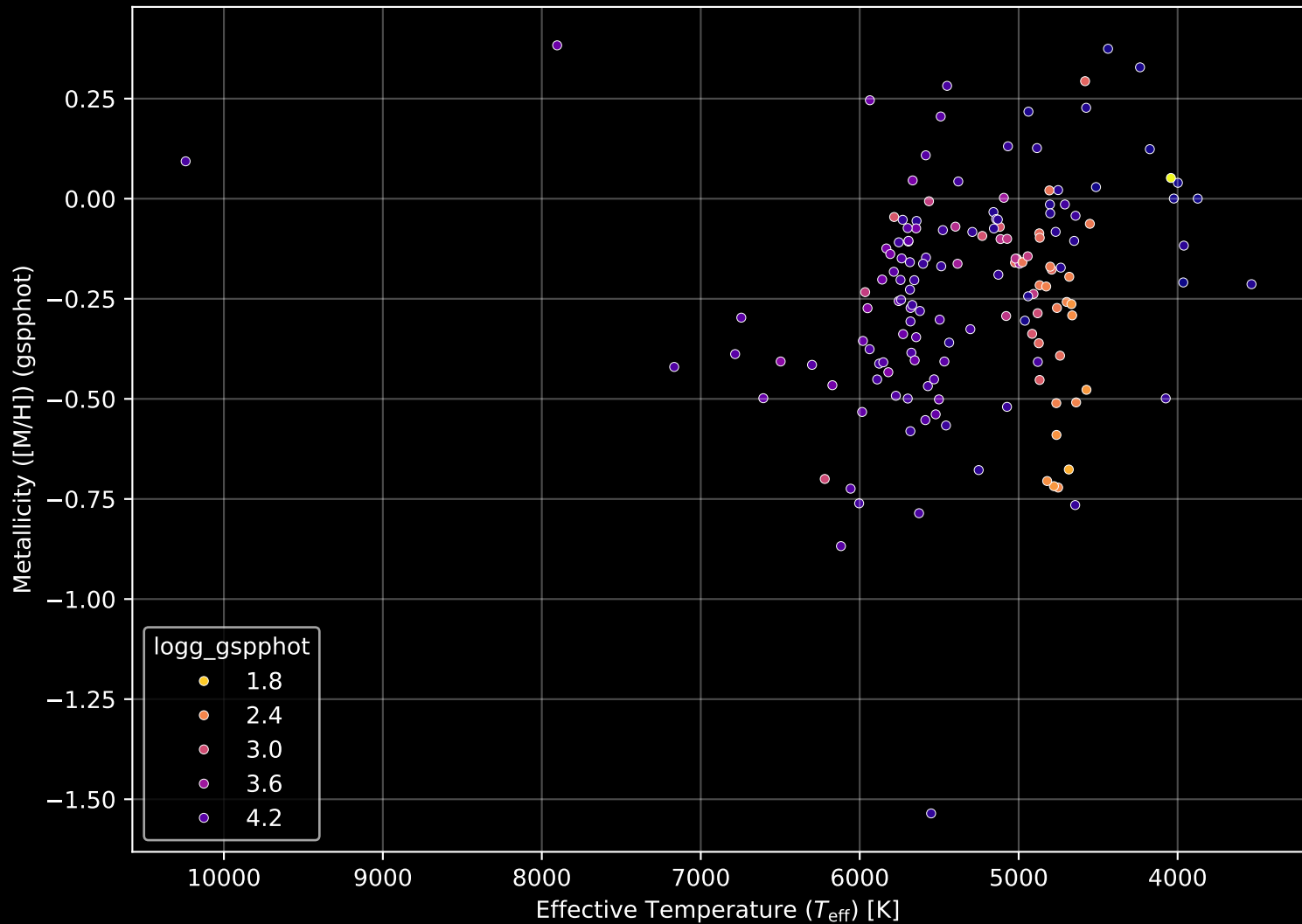
APOGEE DR17 Field: [044+37_MGA] Stellar Population Parameters (n= 153)
