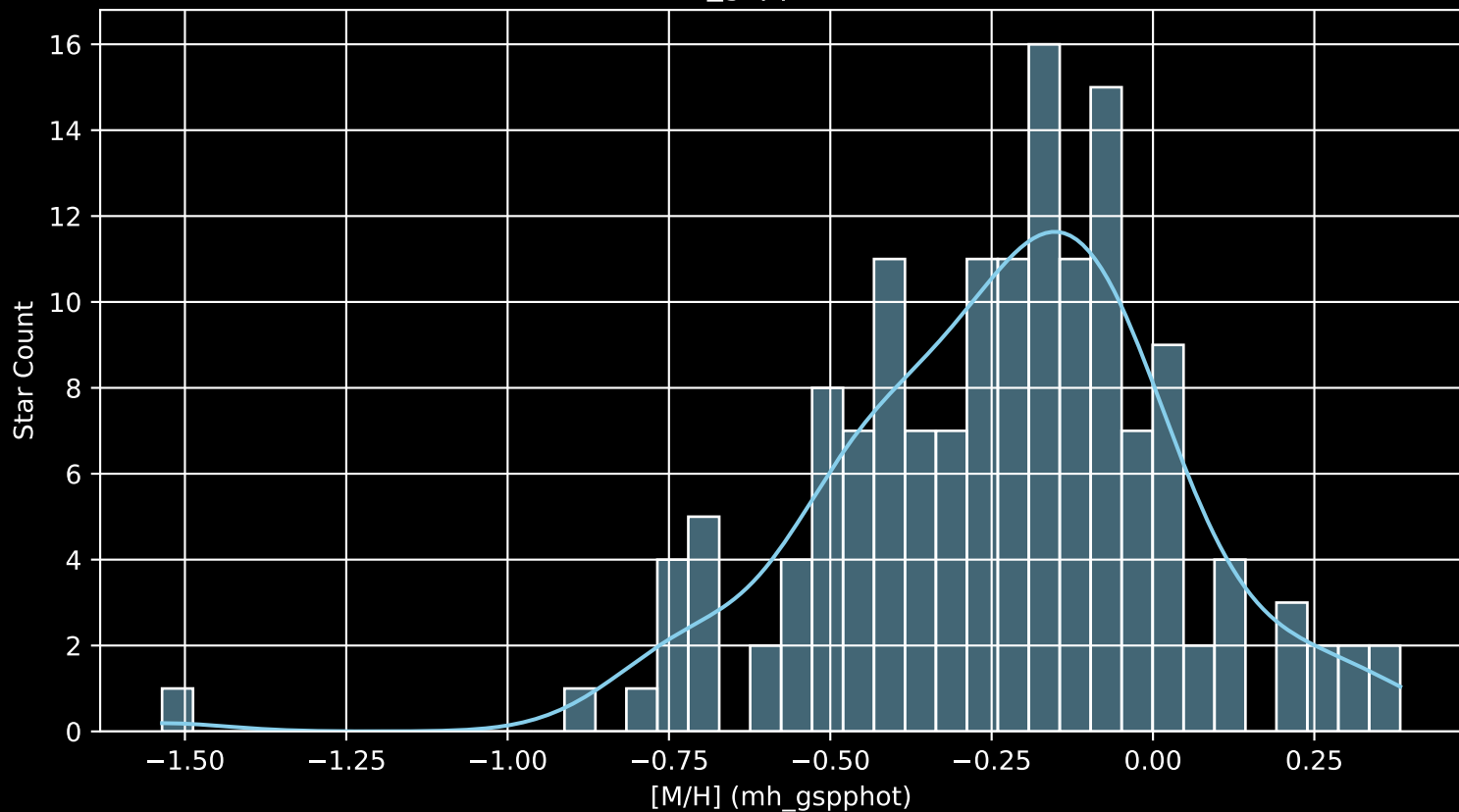
APOGEE DR17 Field: [044+37_MGA [M/H] (mh_gspphot) (n= 153)
